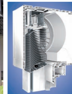
Aufsatzkasten mit Raffstore
